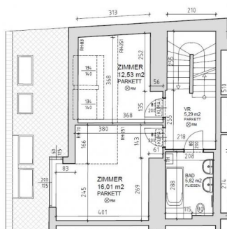
2. DACHGESCHOSS
