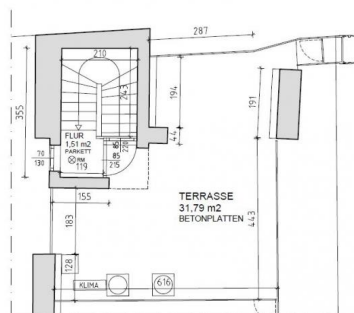
DACHDRAUFSICHT
