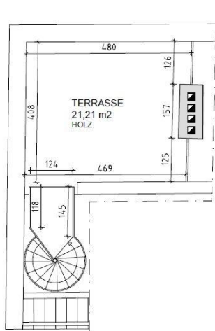
DACHDRAUFSICHT
