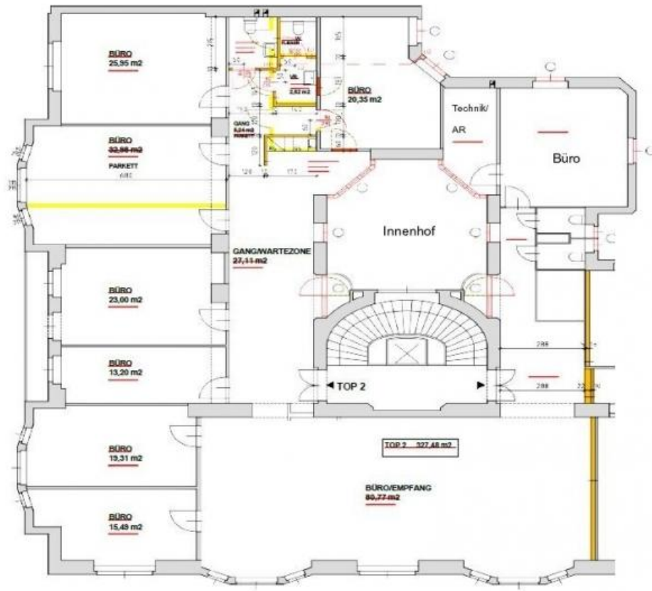
1.OBERGESCHOSS M 1:100
