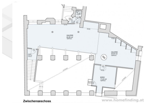
Zwischenegeschoss
